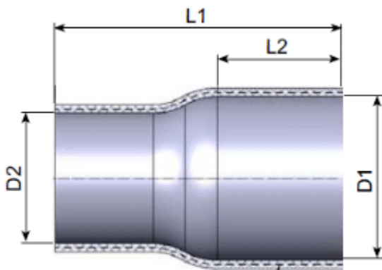
1074593 Sisä Ø 45/55, L1 75/L2 35-40 mm EPDM - VAHVIKK. LETKUKARTIO
