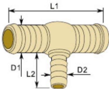
1078517 Ø 10,5/5,0 x 50/17 mm LETKULIITIN T-KAPPALE, TERÄS
