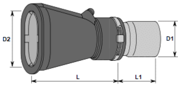
1078611 D1 63 mm/D2 70-110 mm PAKOKAASULETKUKARTIO
